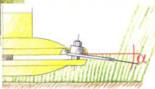
Patentově chráněný disk a uložení nože pro dosažení rovnoměrné výšky strniště
