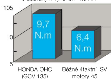
Srovnání krouticího momentu u motorů s udávaným výkonem 4,5 HP.
