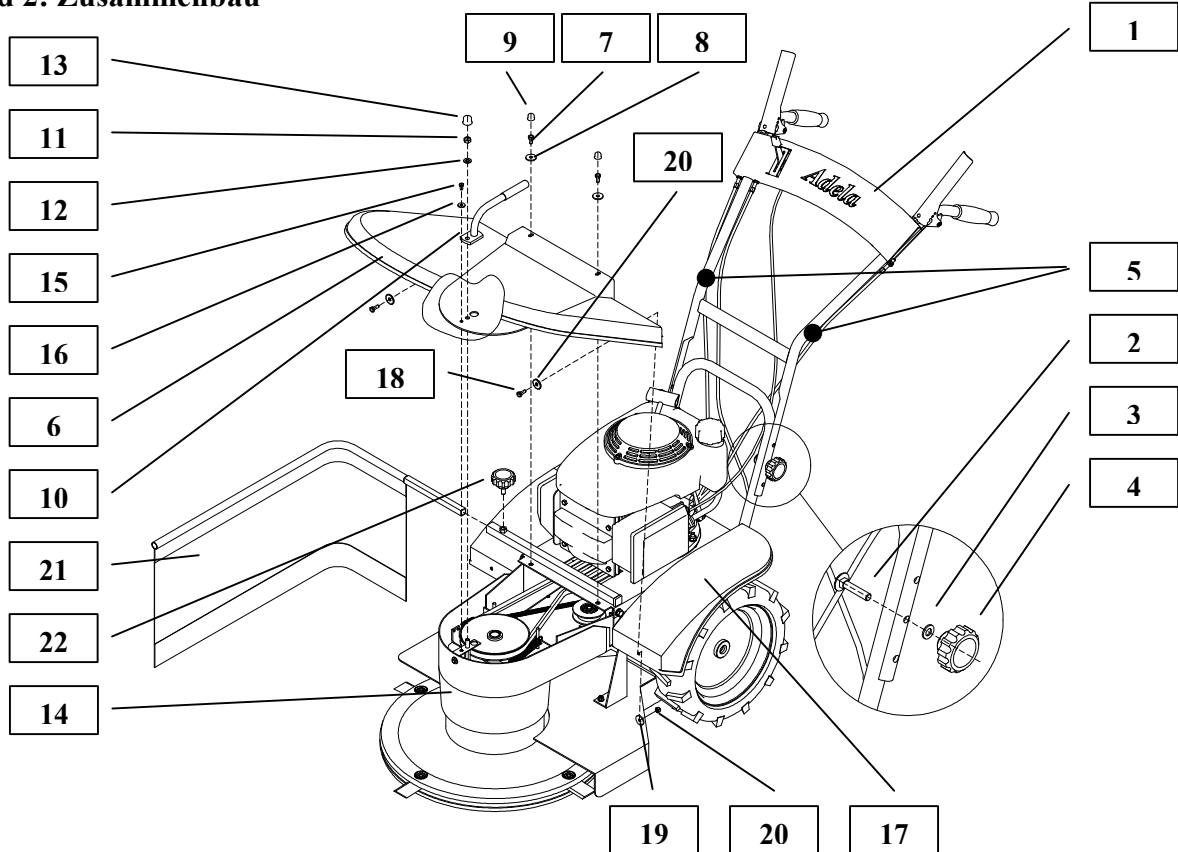
Bild 2: Zusammenbau
