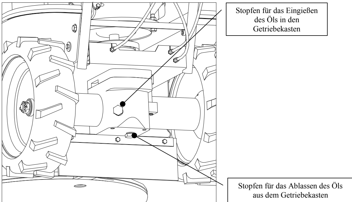
Bild 4: Ölstopfen
