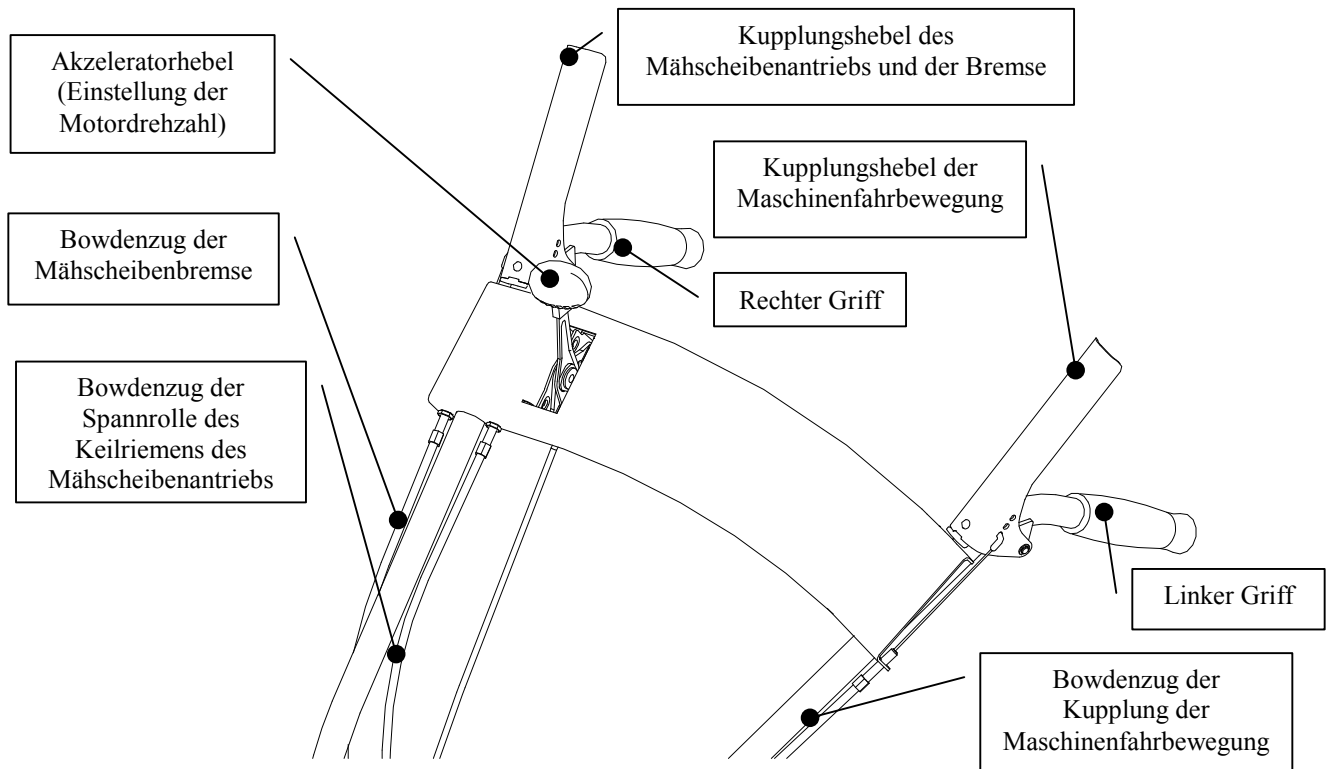
Bild 3: Lenkholme und Akzeleratorhebel
