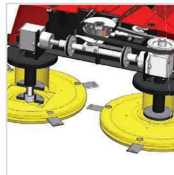
ŘEZ POHONU
