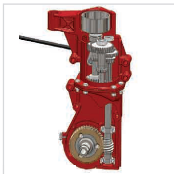
PRŮŘEZ PŘEVODOVÝCH SKŘÍNÍ DSK-317 A DSK-316
