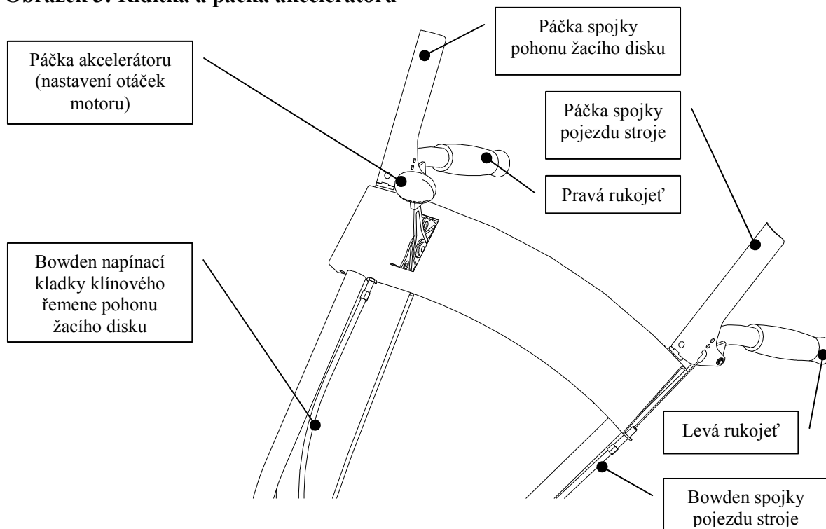
Obrázek 3: Řídítka a páčka akcelérátoru
