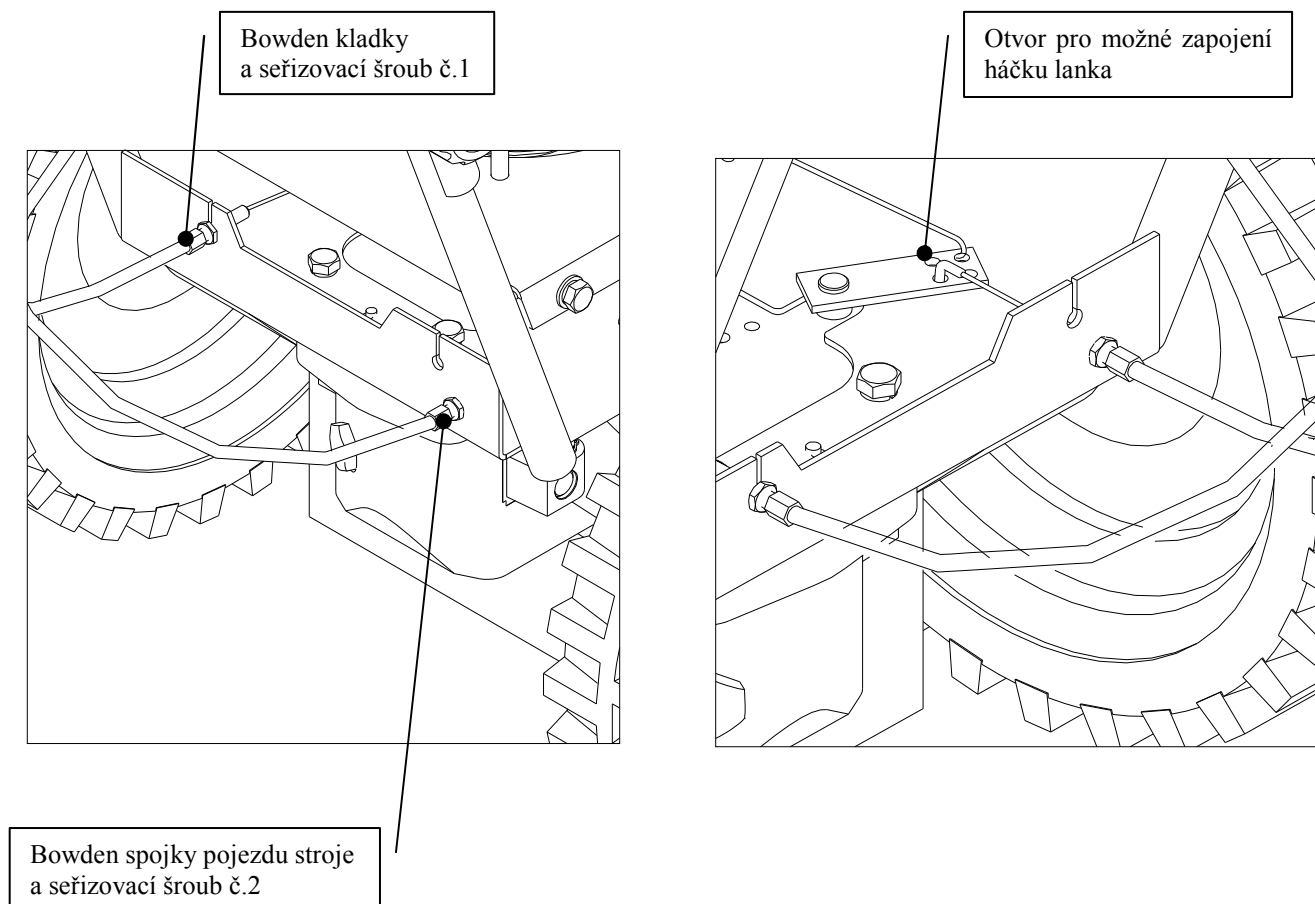
Obrázek 8: Bowdeny a seřizovací šrouby
