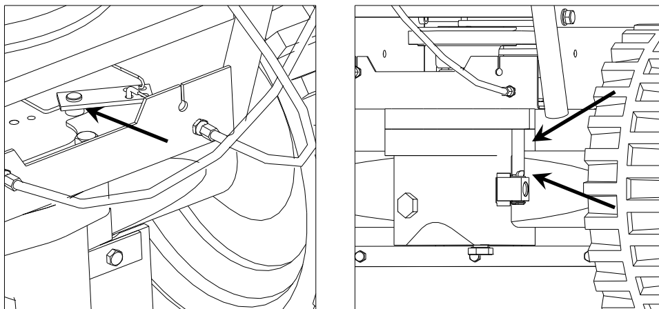
Obrázek 5.2: Čep ramene napínací kladky
