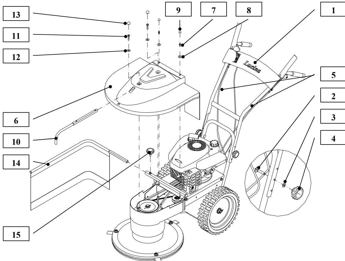
Obrázek 2: Sestavení stroje
